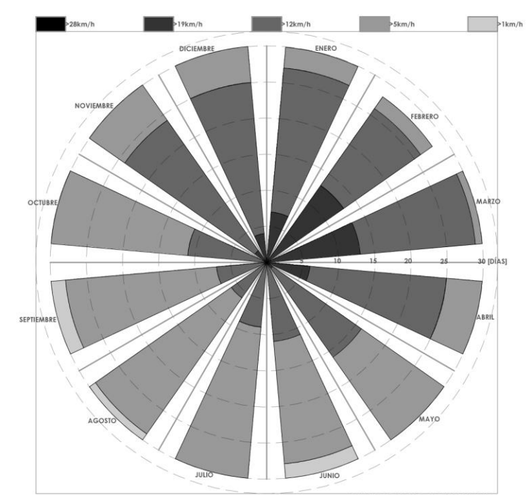
DIAGRAMA DE VIENTO REGISTRO DE VELOCIDADES MEDIAS POR NÚMERO DE DÍAS Y AÑO
