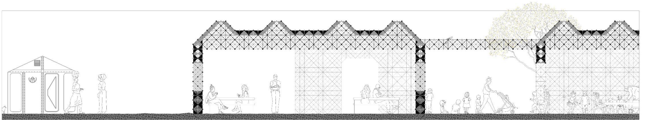
SECCIÓN B-B ESCALA 1_50.
