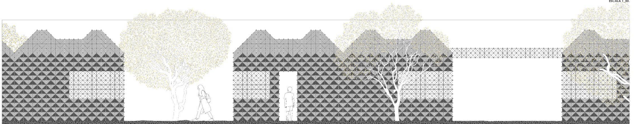
SECCIÓN E-E ESCALA 1_50.
