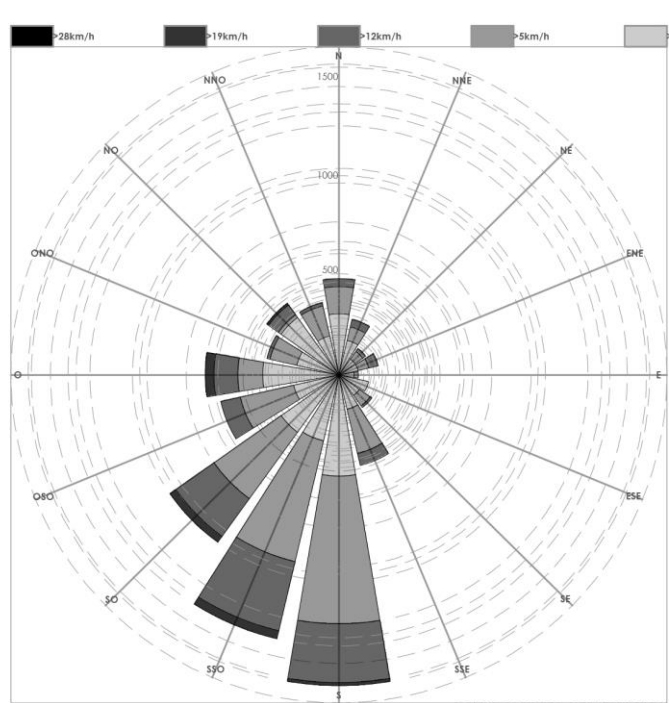
DIAGRAMA DE VIENTO DIRECCIÓN E INTENSIDAD DE VIENTOS POR HORAS ANUALES EN BRIA
