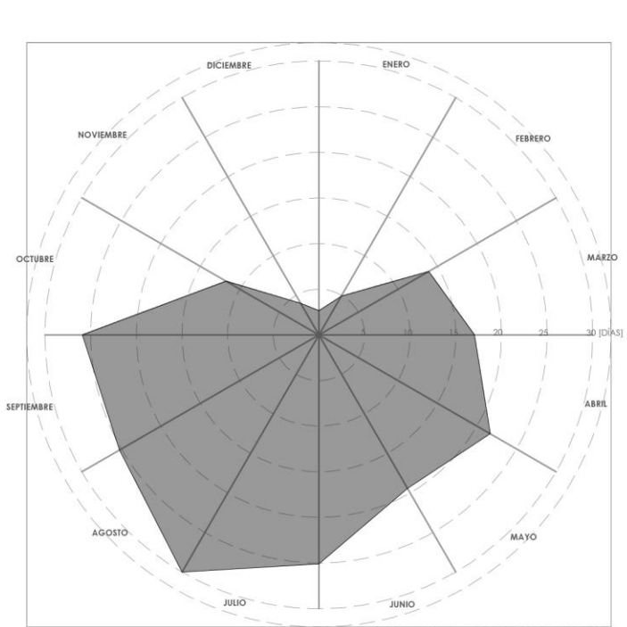
DIAGRAMA DE PRECIPITACIONES NÚMERO DE PRECIPITACIONES POR MES AL AÑO
