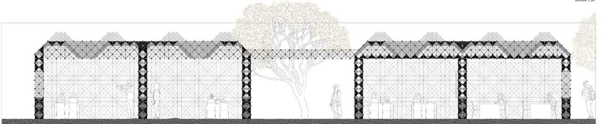
SECCIÓN C-C ESCALA 1_50.
