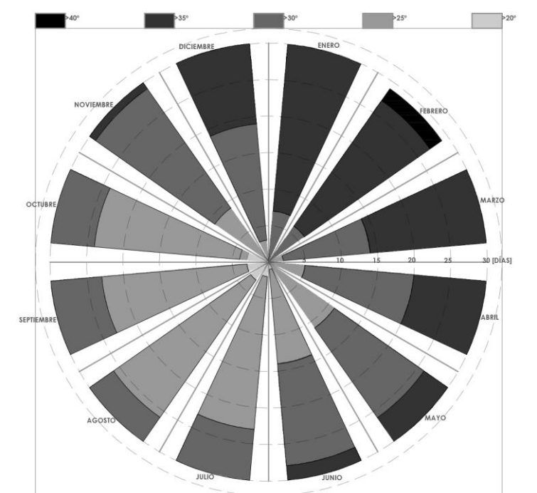
DIAGRAMA DE TEMPERATURAS REGISTRO DE TEMPERATURAS MÁXIMAS POR NÚMERO DE DÍAS Y AÑO
